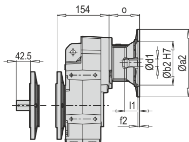
D/M 302 - 303 B5 PAM B5/B14
