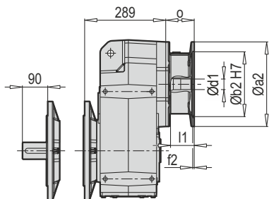
D/M 602 - 603 B5 PAM B5/B14
