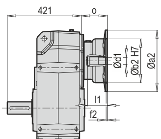
M 702 - 703 PAM B5/B14
