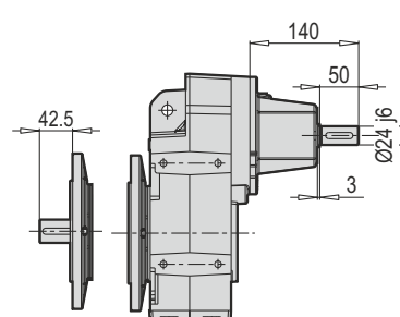
D/M 302 - 303 B5 W
