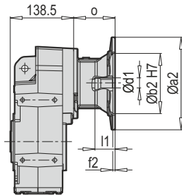
D 302 - 303 PAM B5/B14
