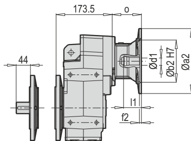
D/M 352 - 353 B5 PAM B5/B14
