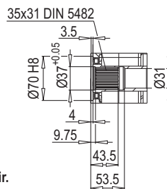
A DETAYI
