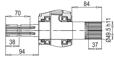
6 DIN 9611 1"3/8 Z6 DIN 5482 50x45
