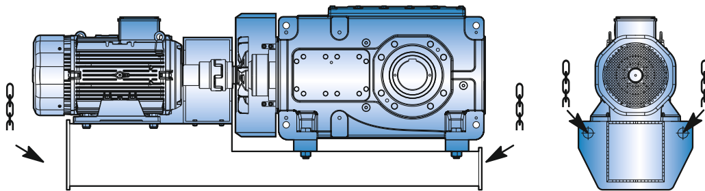
Abbildung 2 - d: Positionen der zusätzlichen Hebeunkte für Getriebe mit Drehmomentstütze des Typs PB
