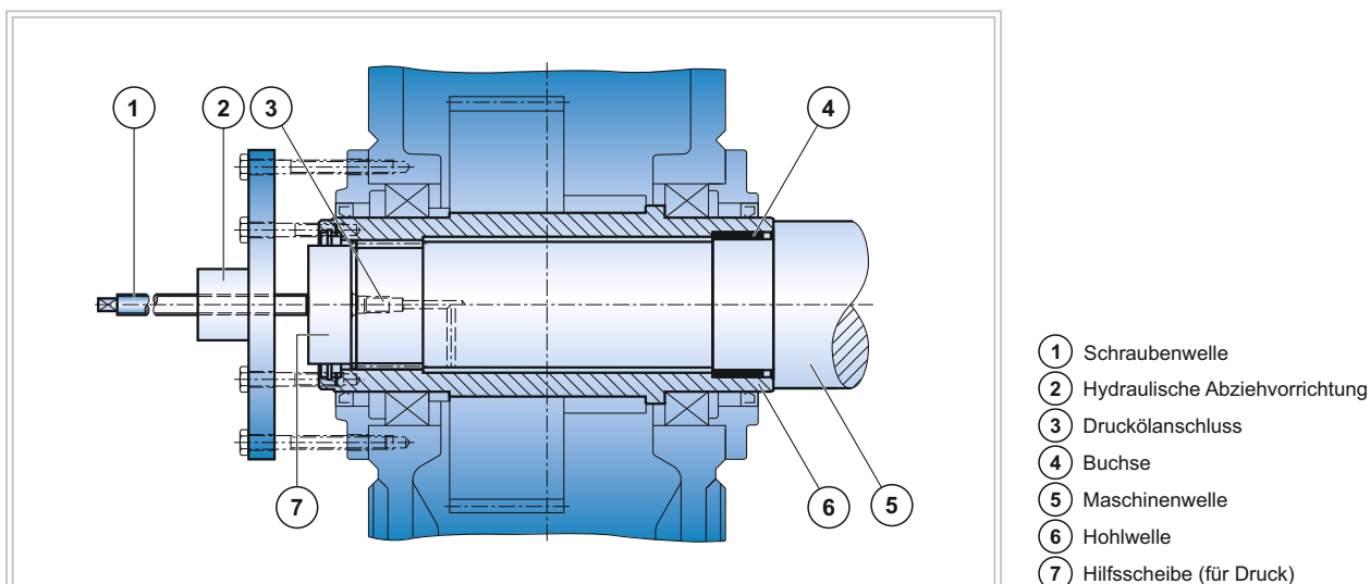
Abbildung 51: Demontage mit hydraulischer Abziehvorrichtung
