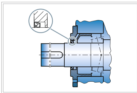
Abbildung 13: Labyrinthdichtung
