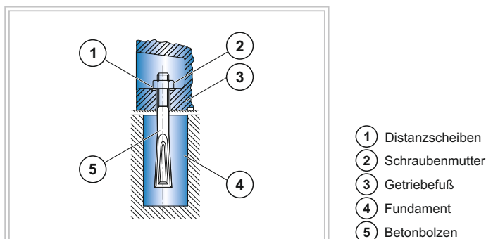
Abbildung 36: Betonbolzen
