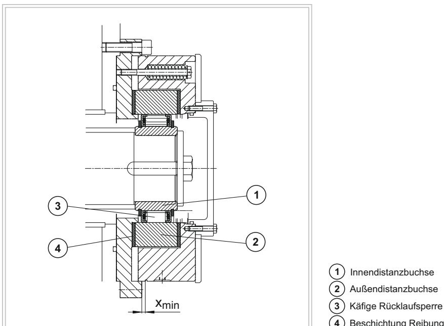
Abbildung 18: Rücklaufsperre mit Drehmomentbegrenzung
