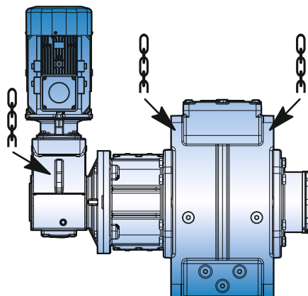
Abbildung 2 - e: Positionen der zusätzlichen Hebeunkte für Hilfsantriebsgetriebe des Typs PB / PH
