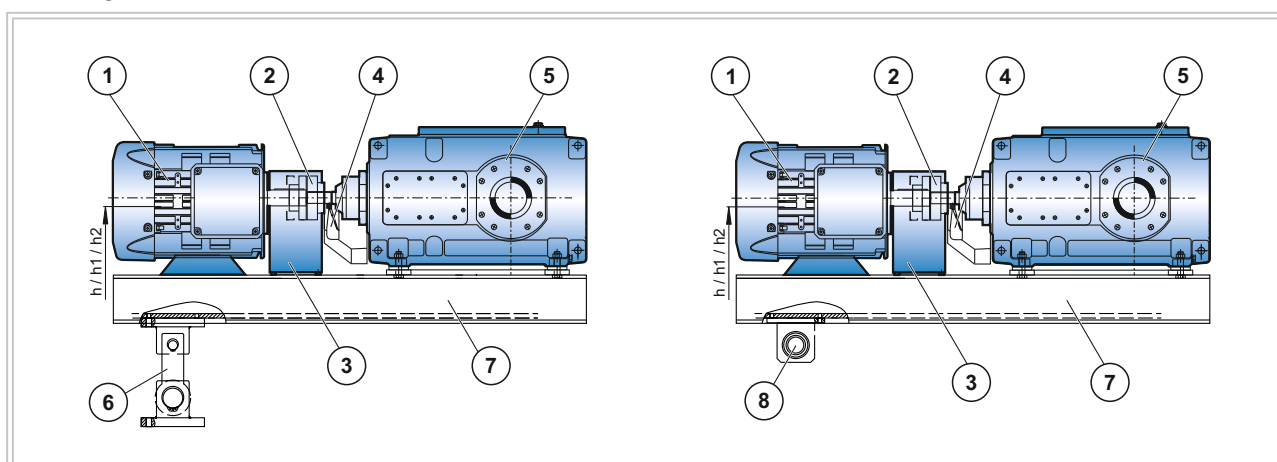
Abbildung 40: Drehmomentstütze für Getriebe
