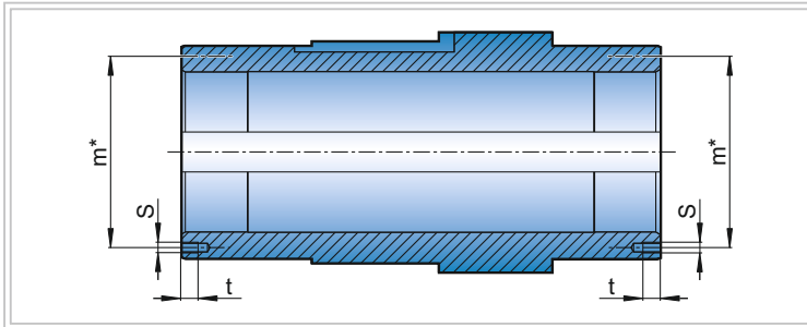
Abbildung 47: Hohlwelle mit Passfeder
