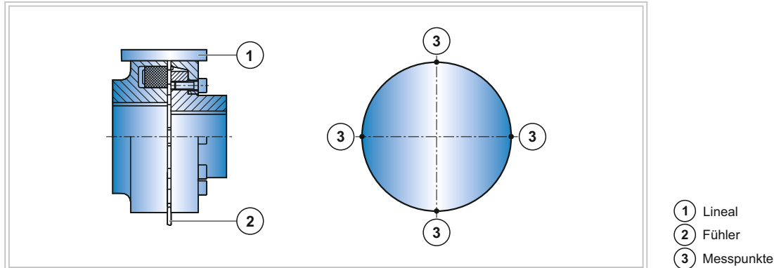
Abbildung 54: Ausrichtungsprozess mit flexibler Kupplung
