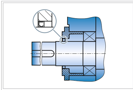
Abbildung 12: Drehwellendichtung
