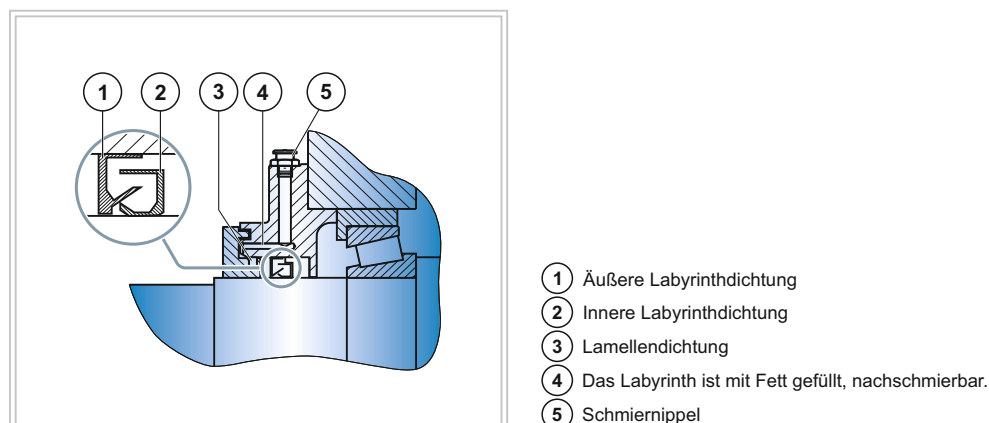
Abbildung 16: Tacolab-Dichtung
