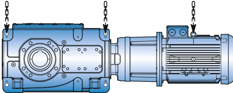
Abbildung 2 - c: Positionen der zusätzlichen Hebeunkte für Getriebemotoren des Typs PB
