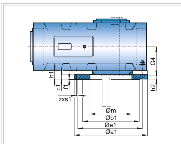
Abbildung 41: Blockflanschgetriebe
