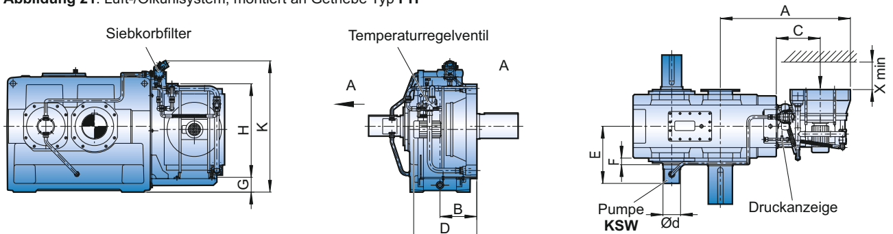
Abbildung 21: Luft-/Ölkühlsystem, montiert an Getriebe Typ PH
